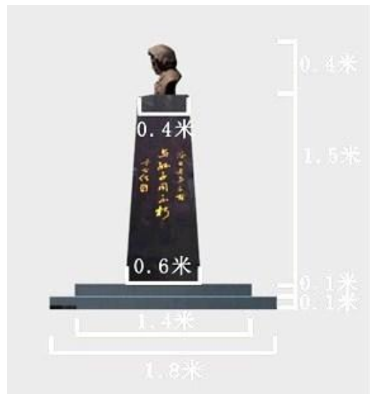
右面設計圖
