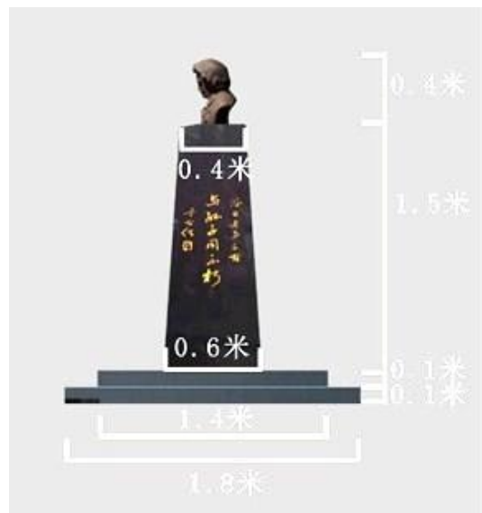
右面设计图
