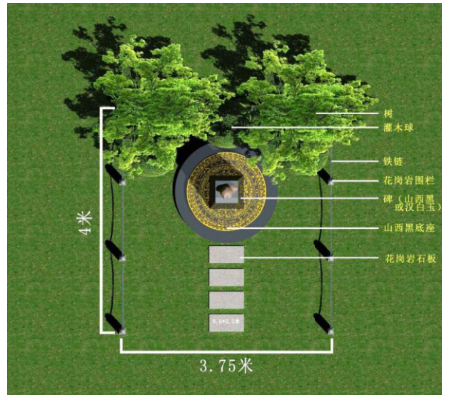
鸟瞰设计图
